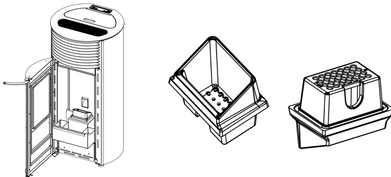
Afbeelding 34. Onderdelen voor dagelijkse en wekelijkse schoonmaak
